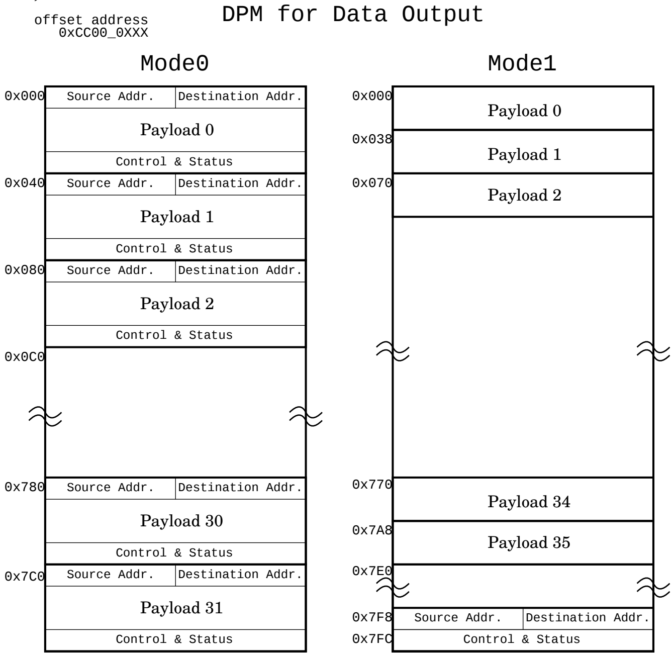
図 23.13: DPM for Data Output
