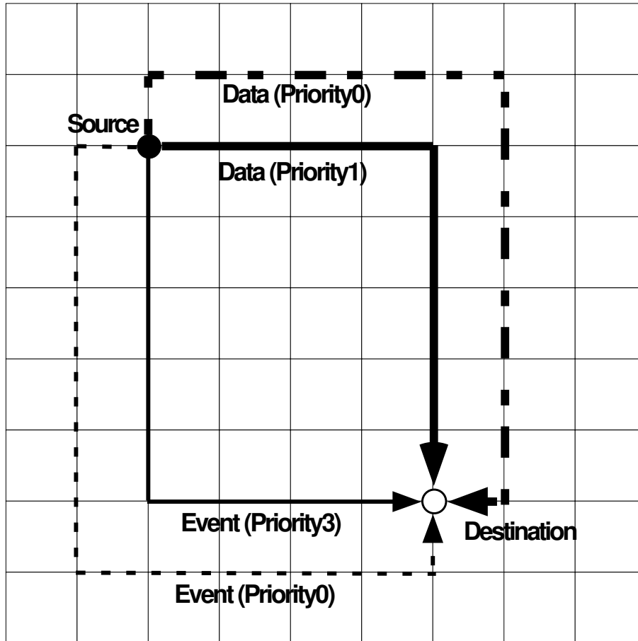
図 23.7: Responsive Link の優先度付経路
