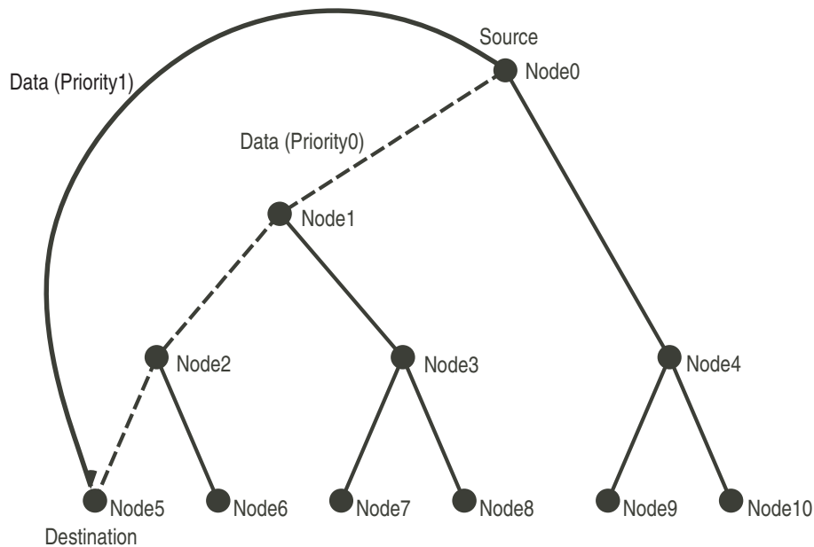
図 23.8: Responsive Link の優先度付木構造経路
