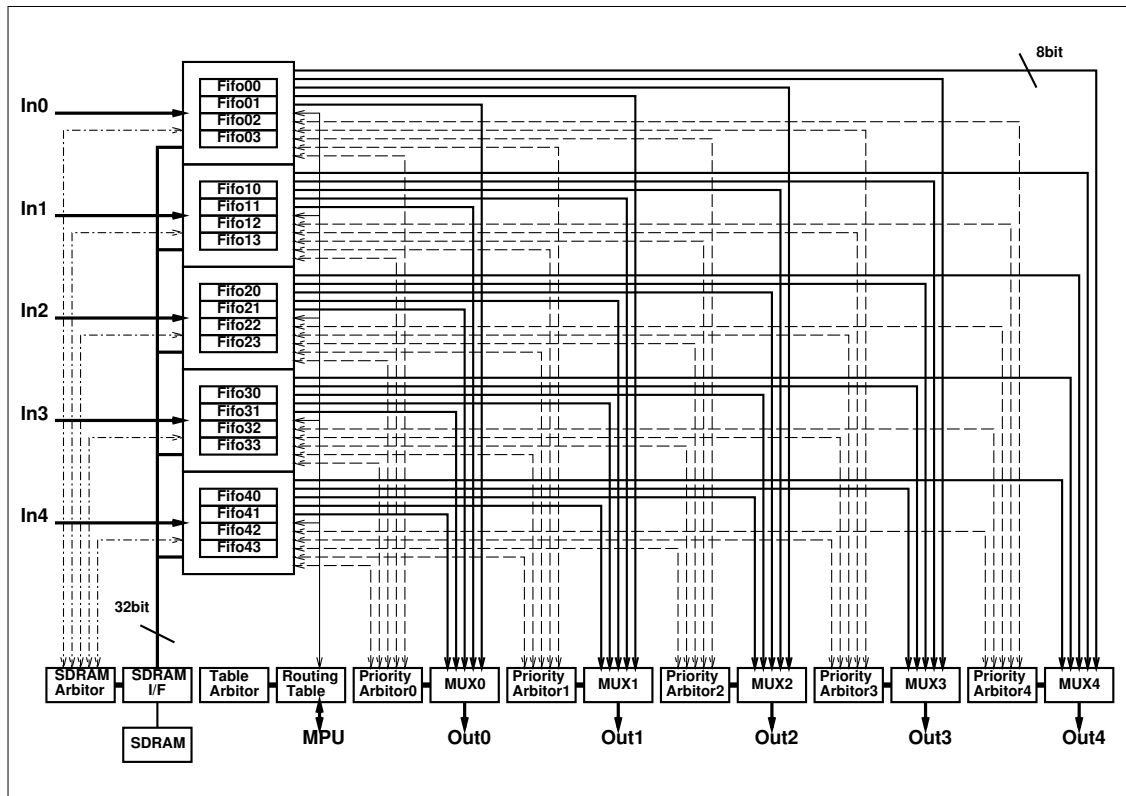
図 23.4: Responsive Link のネットワークスイッチ
