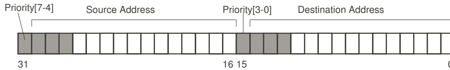
図 23.3: Responsive Link のヘッダフォーマット
