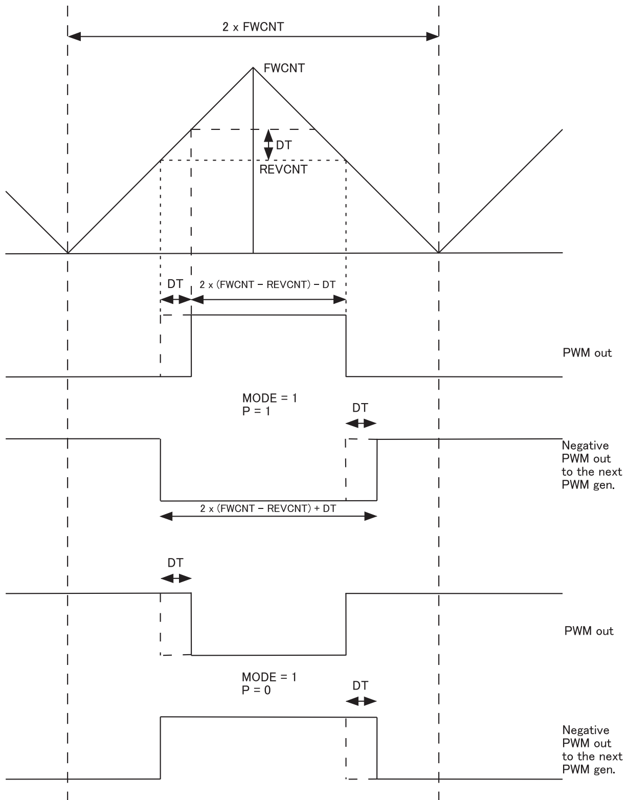
図 16.2: 三角波モード
