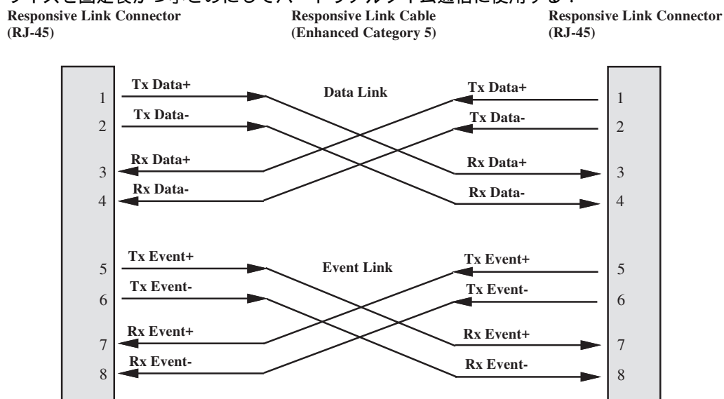
図 23.1: Responsive Link インタフェース
