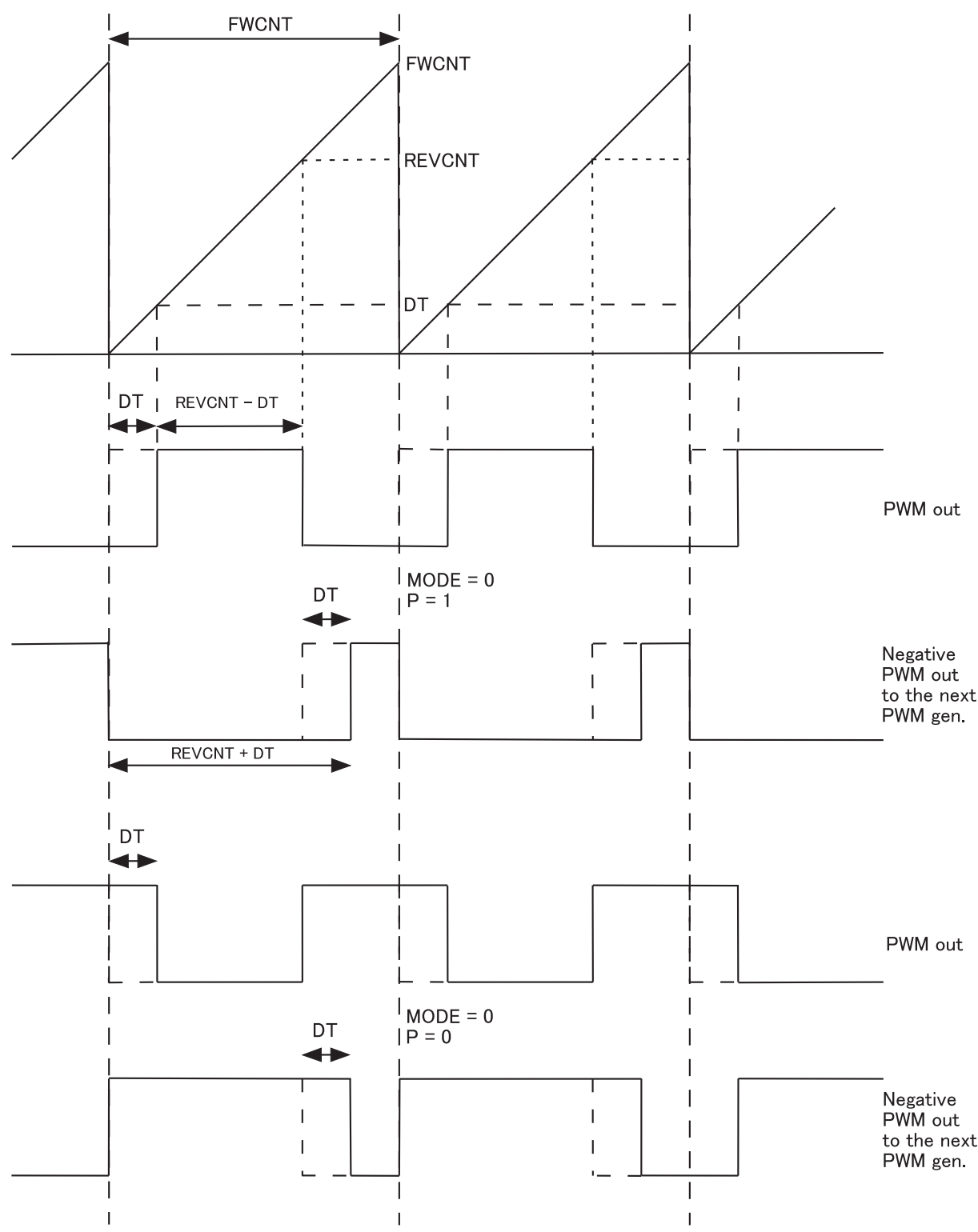
図 16.1: ノコギリ波モード
