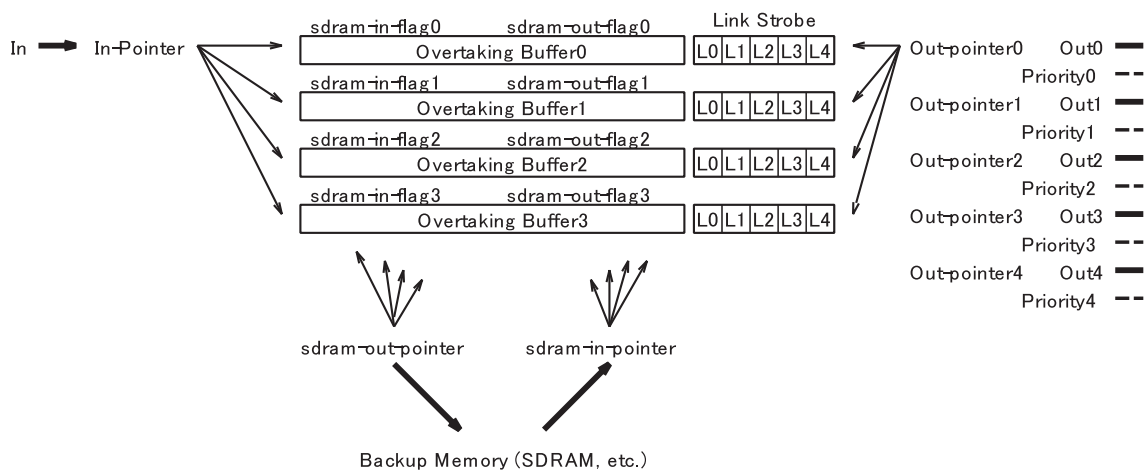
図 23.5: Responsive Link の追い越し用バッファ
