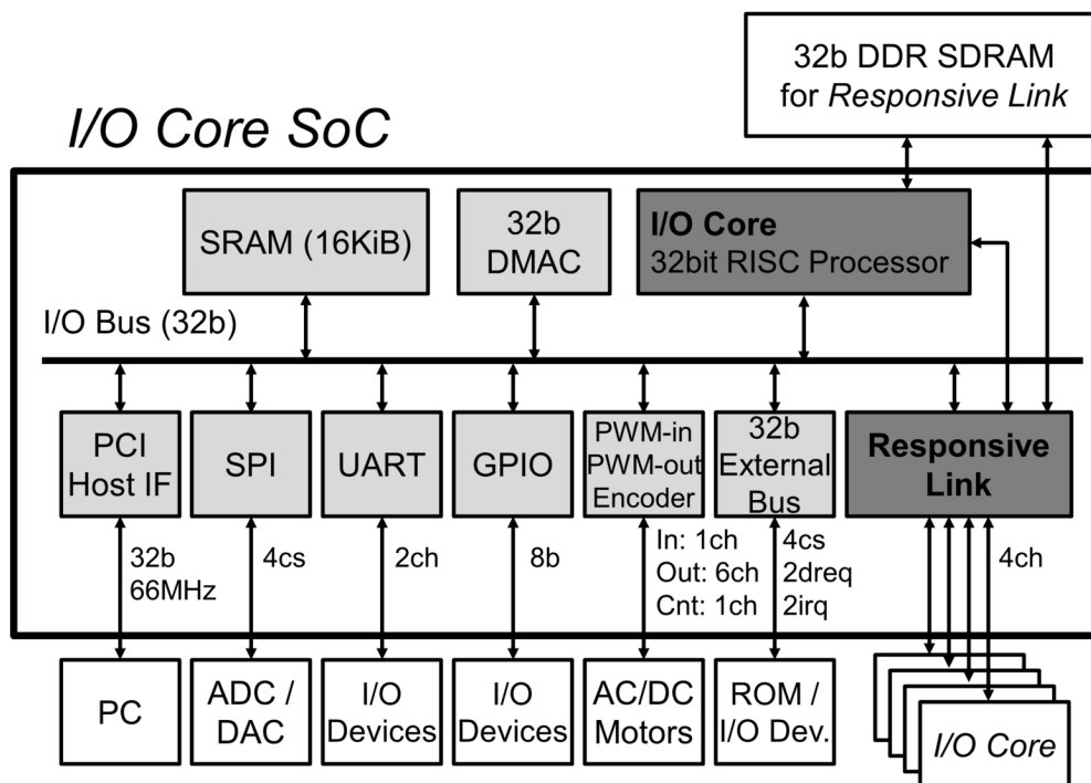
図 1.1: I/O Core のブロック図
