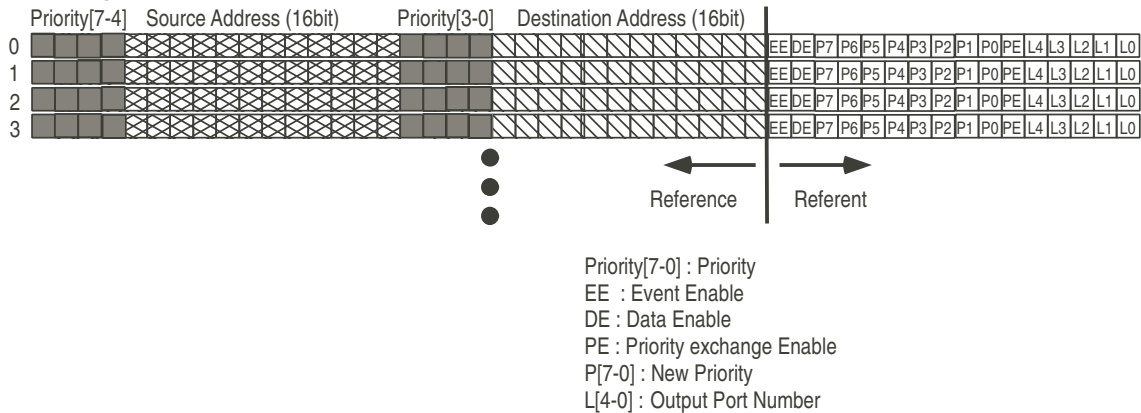
図 23.6: Responsive Link のルーティングテーブル
