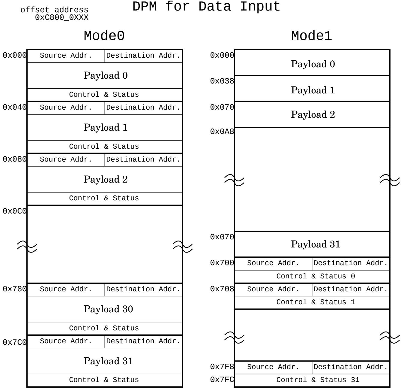
図 23.15: DPM for Data Input
