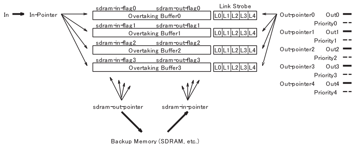
図 26.5: Responsive Link の追い越し用バッファ
