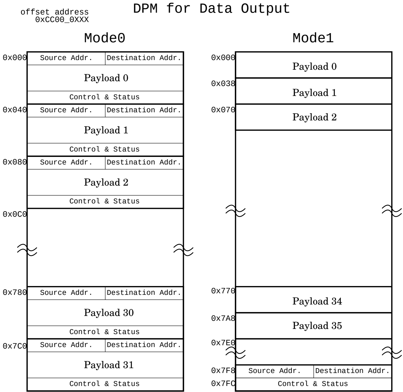
図 26.13: DPM for Data Output
