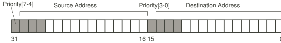
図 26.3: Responsive Link のヘッダフォーマット
