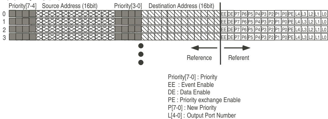
図 26.6: Responsive Link のルーティングテーブル
