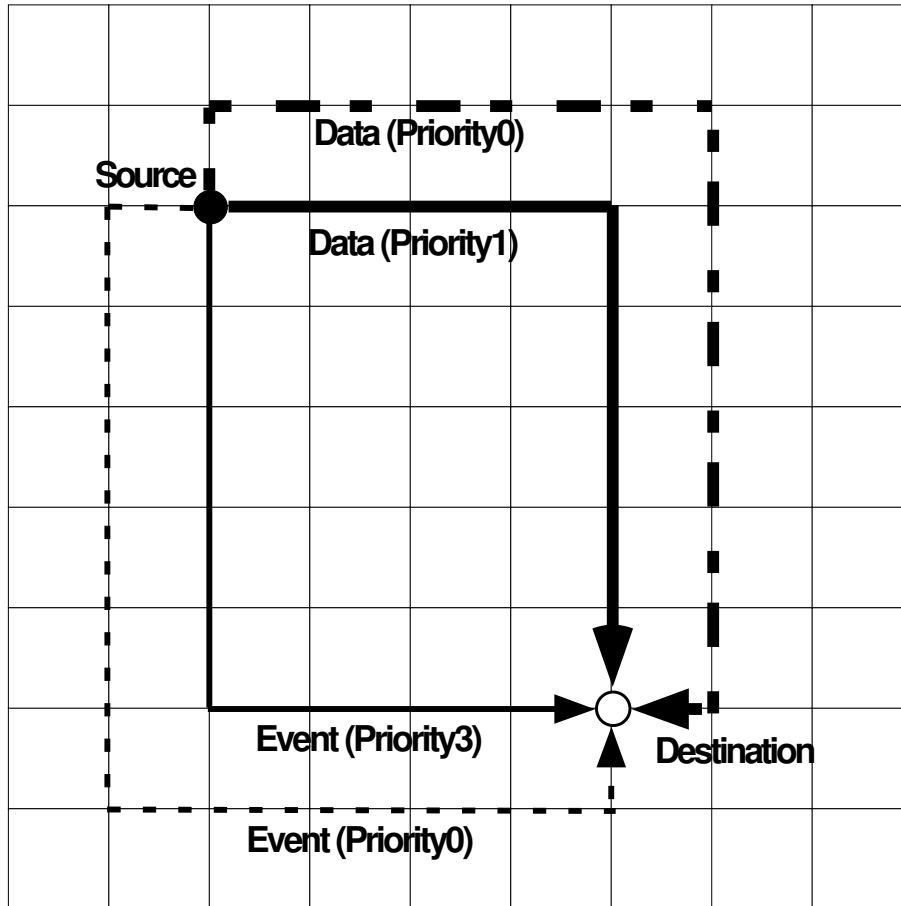
図 26.7: Responsive Link の優先度付経路
