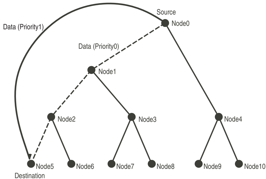
図 26.8: Responsive Link の優先度付木構造経路
