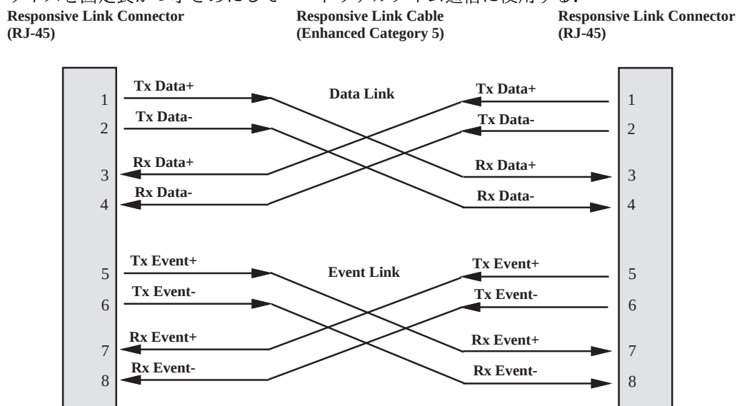
図 26.1: Responsive Link インタフェース
