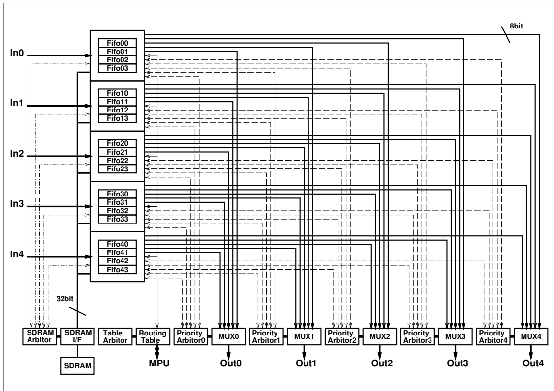
図 26.4: Responsive Link のネットワークスイッチ
