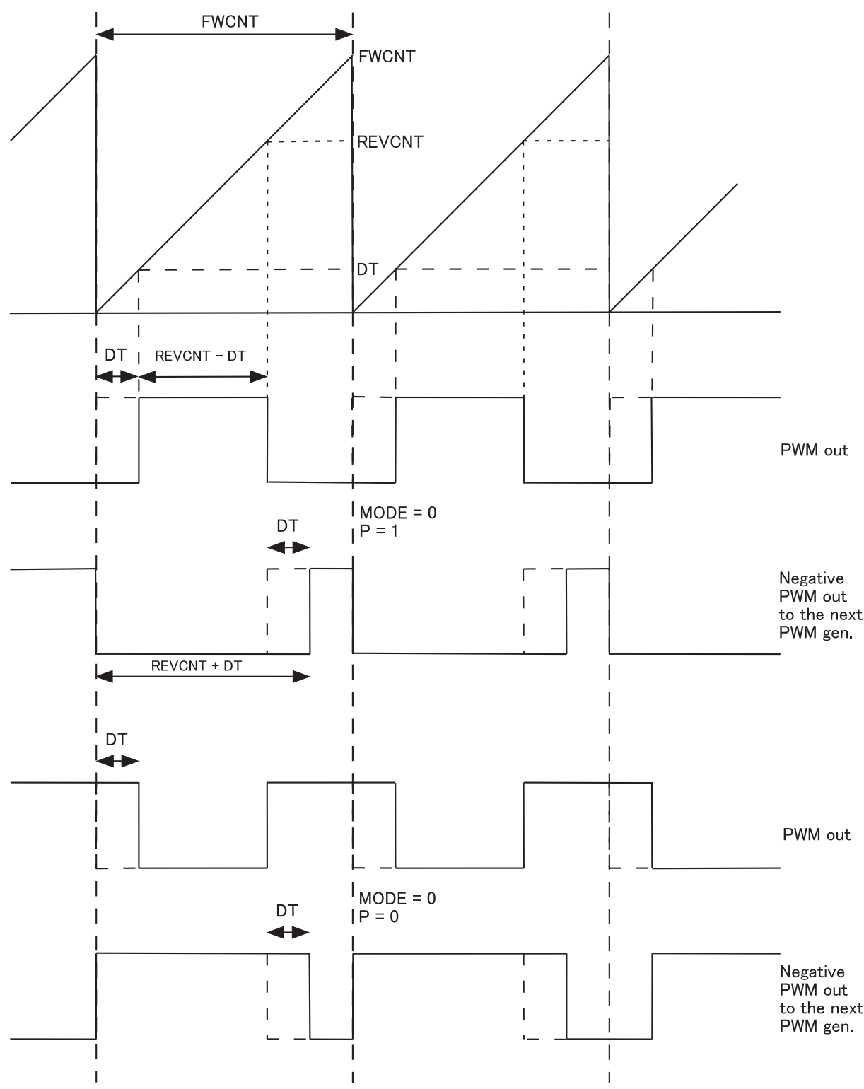
図 17.1: ノコギリ波モード
