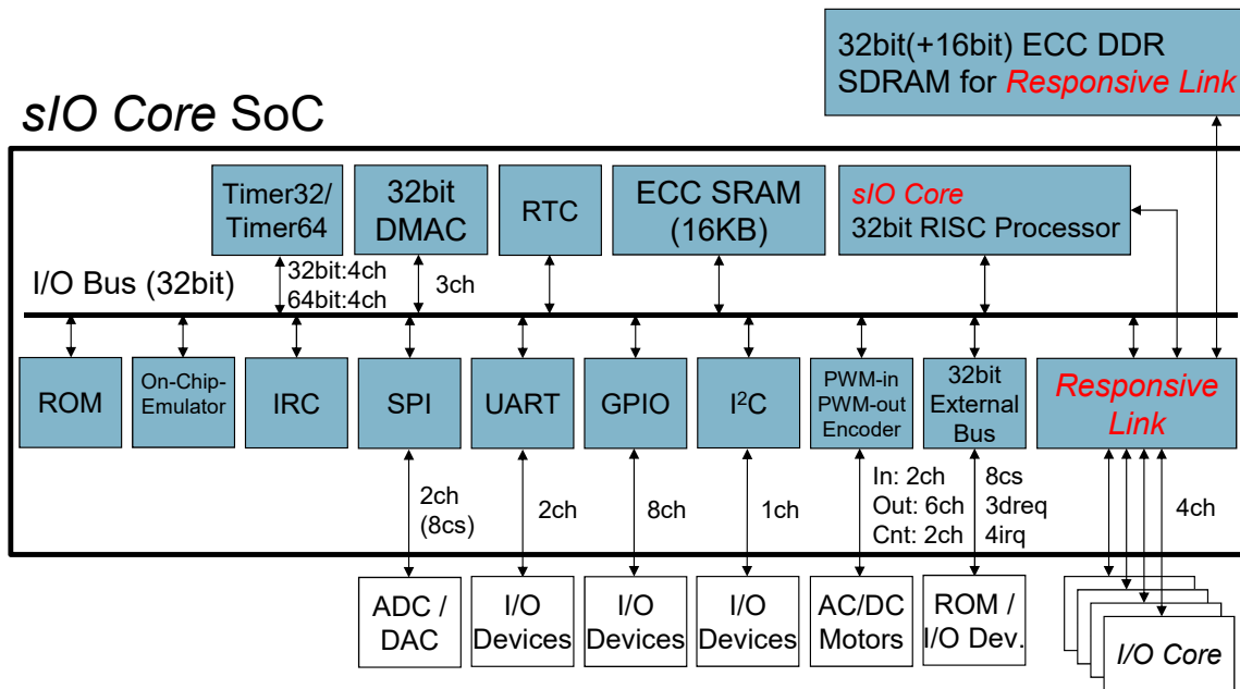
図 1.1: sIO Core のブロック図
